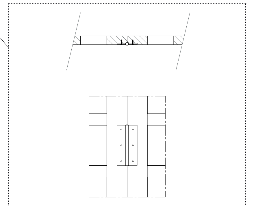
Panneaux liés avec des charnières pour pivoter
